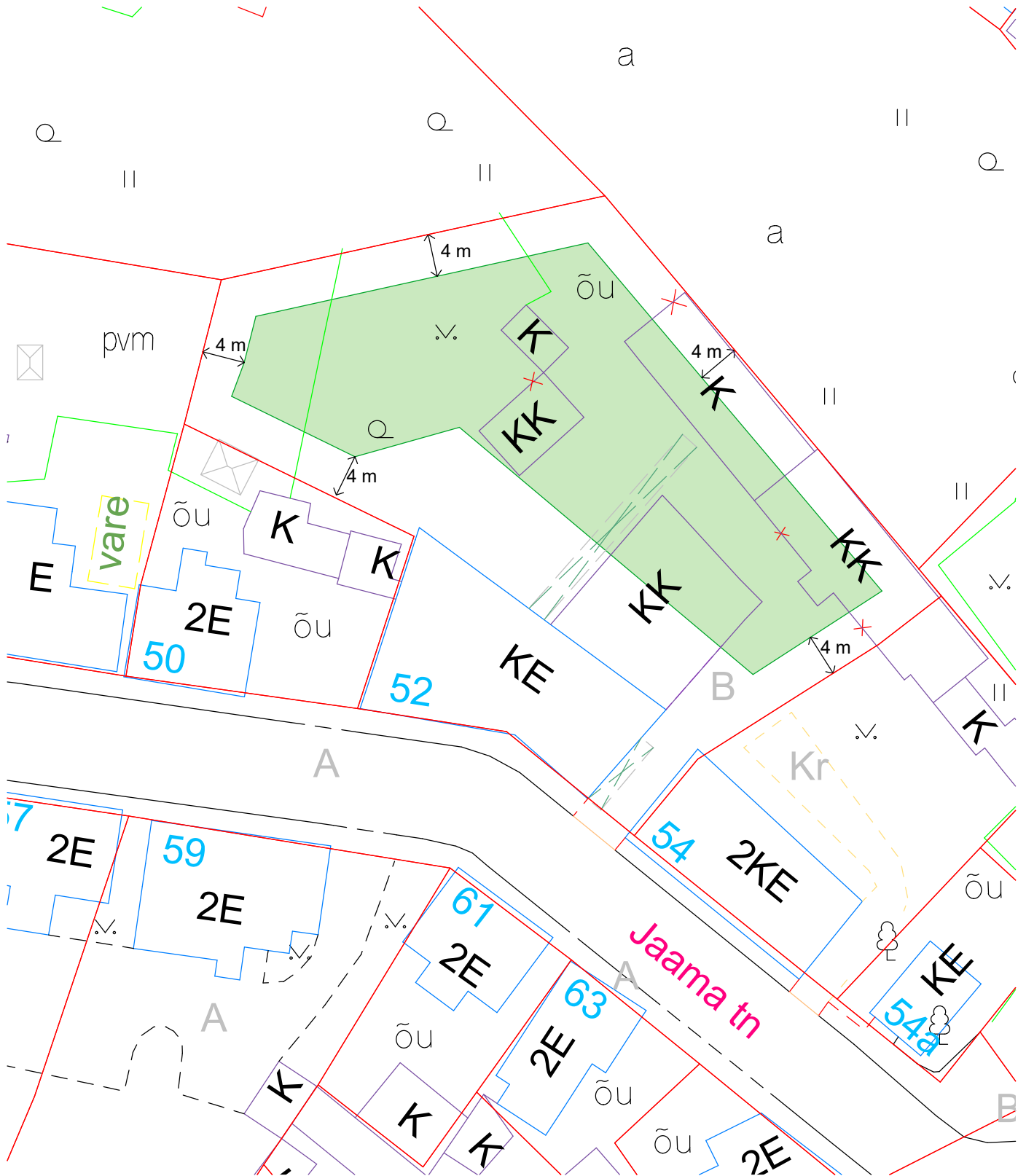
Lisa. Jaama tn 52 ehitusala skeem PTH-21-040
